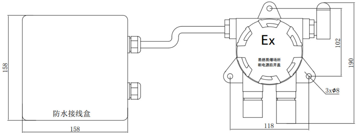
外形结构及尺寸图
